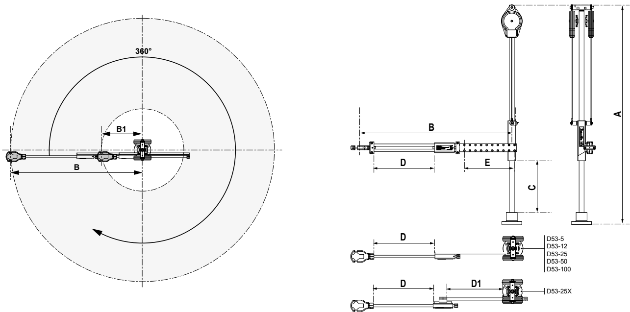
D53 lineal especificacion de producto y area de trabajo
