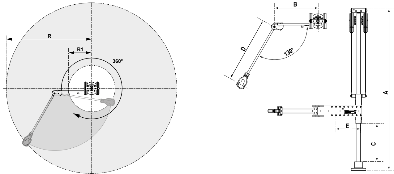
D53 articulado especificaciones y area de trabajo
